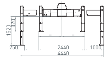
Vierkantabstützung squared outridge
